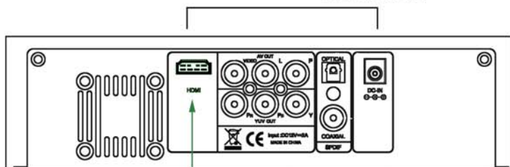
Conexión HDMI
